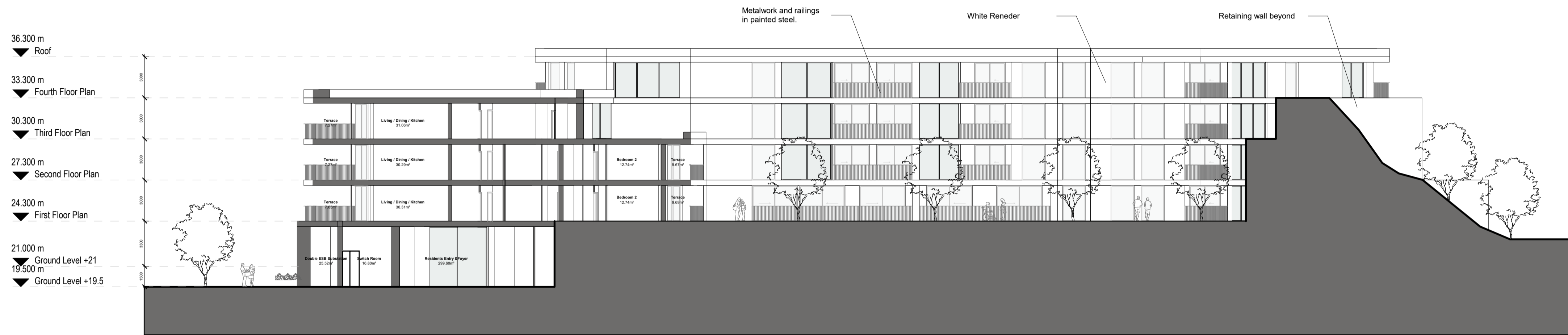
1 Section A-A 1 : 200
